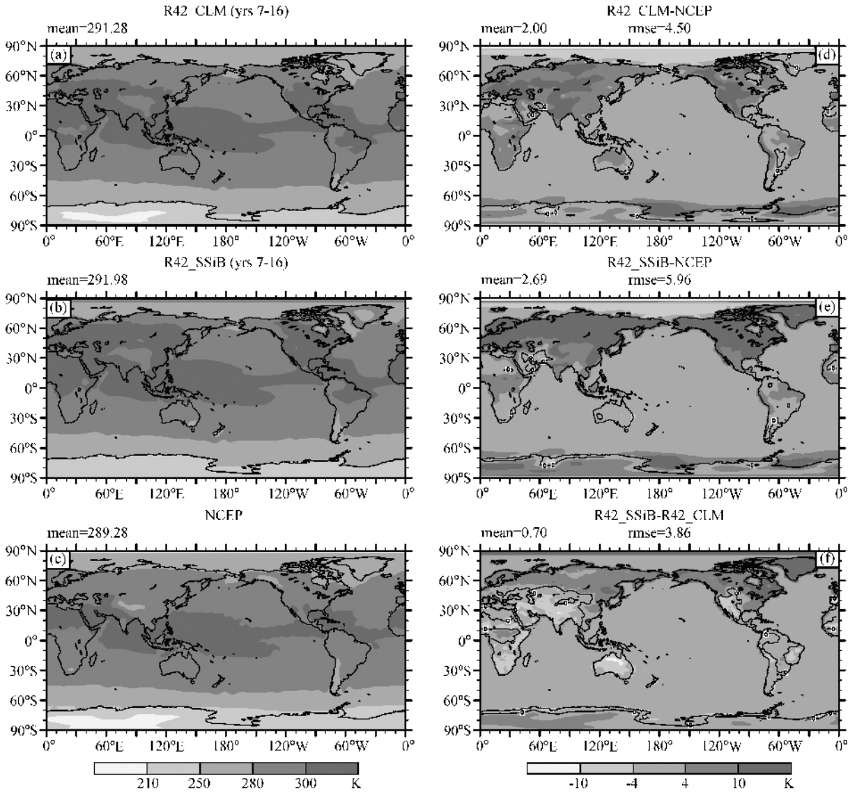
图5 同图2, 但为表面温度
