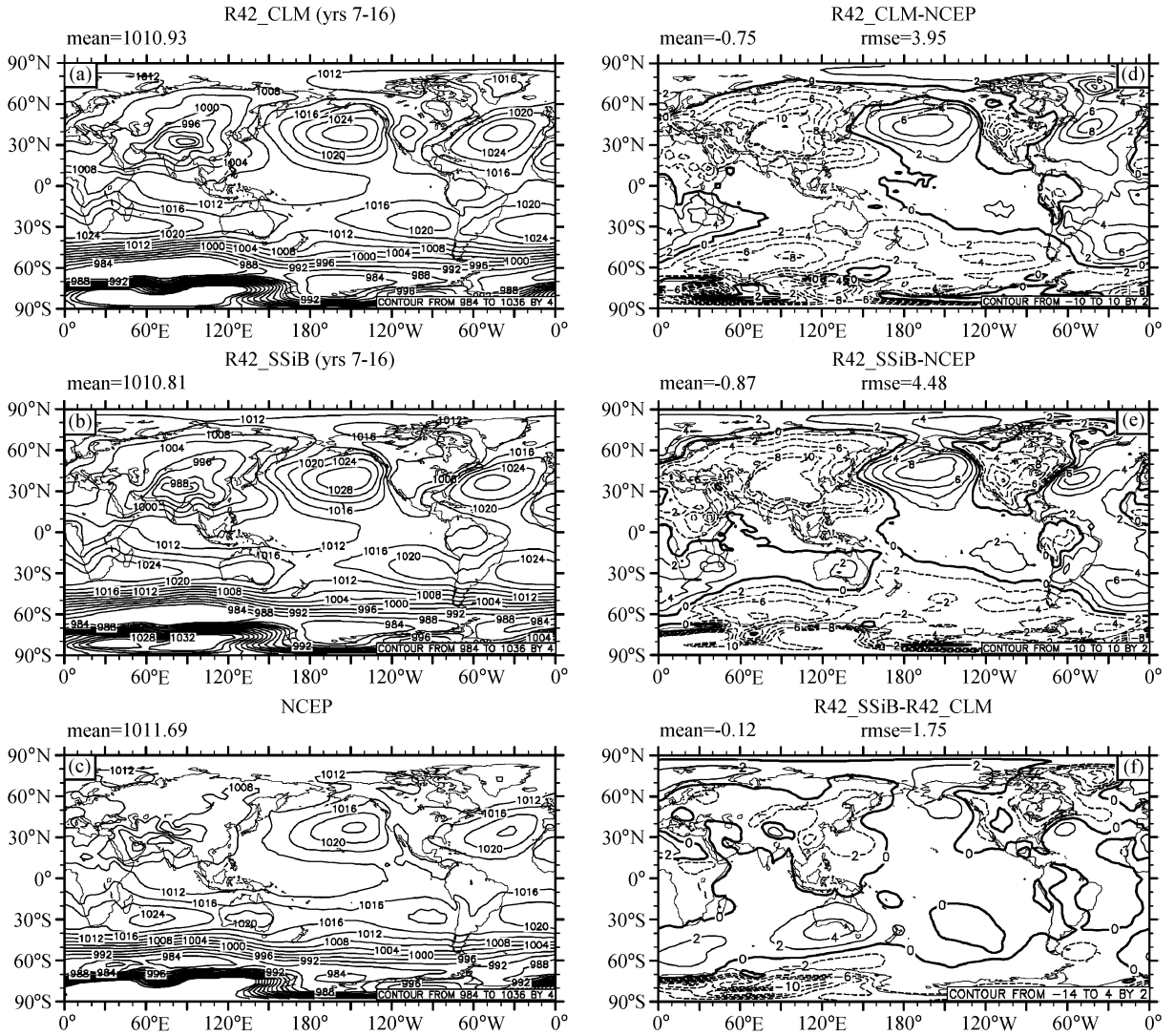
图9 同图2, 但为海平面气压(单位: hPa)
