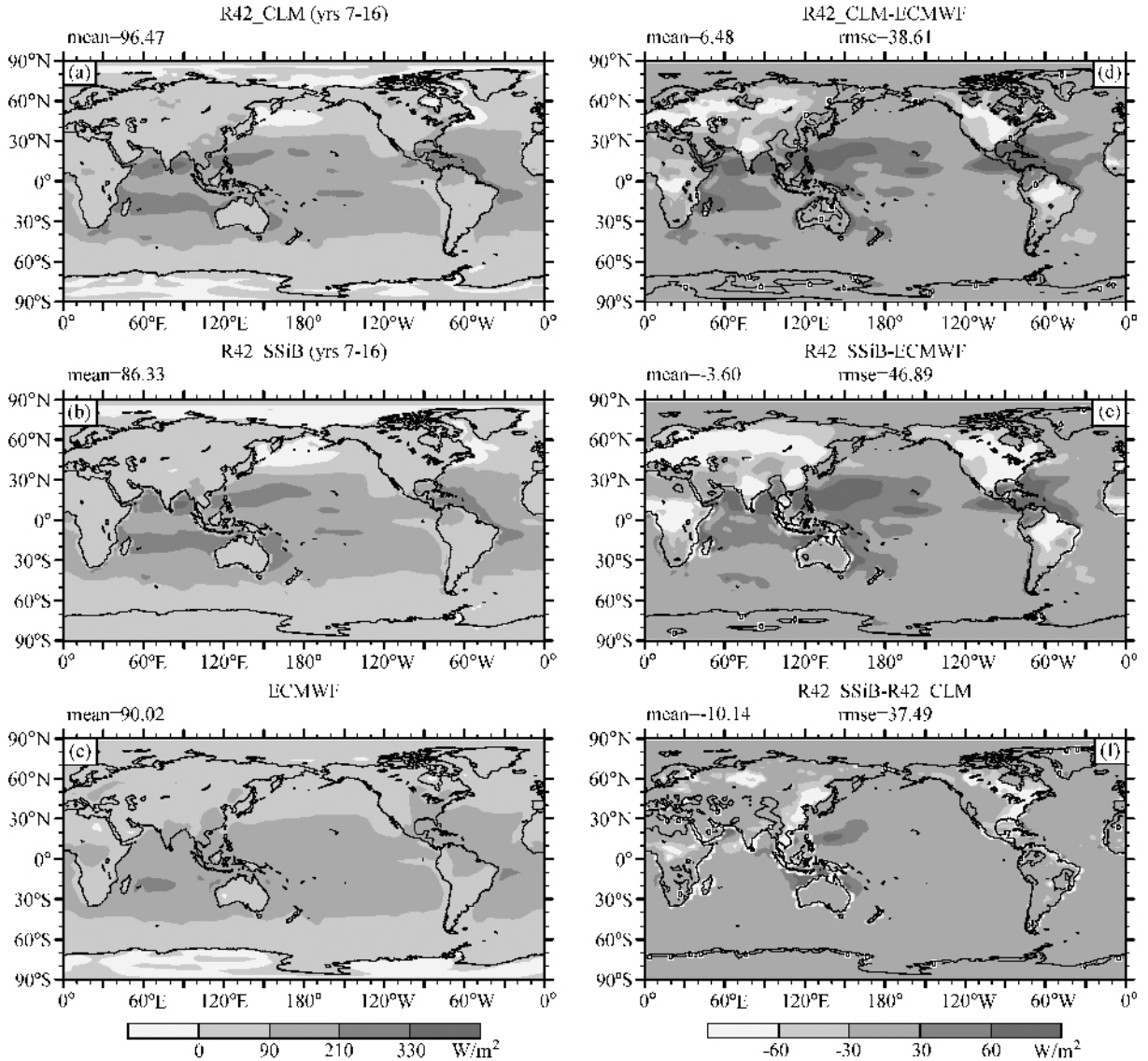
图7 R42_CLM (a)、R42_SSiB (b) 陆气耦合模式模拟和 ECMWF 再分析 (c) 6~8 月 (JJA) 平均表面潜热通量的全球平均分布以及它们之间的差异分布: (d) R42_CLM 与 ECMWF 再分析资料的差异; (e) R42_SSiB 与 ECMWF 再分析资料的差异; (f) R42_SSiB 与 R42_CLM 模式模拟差异
