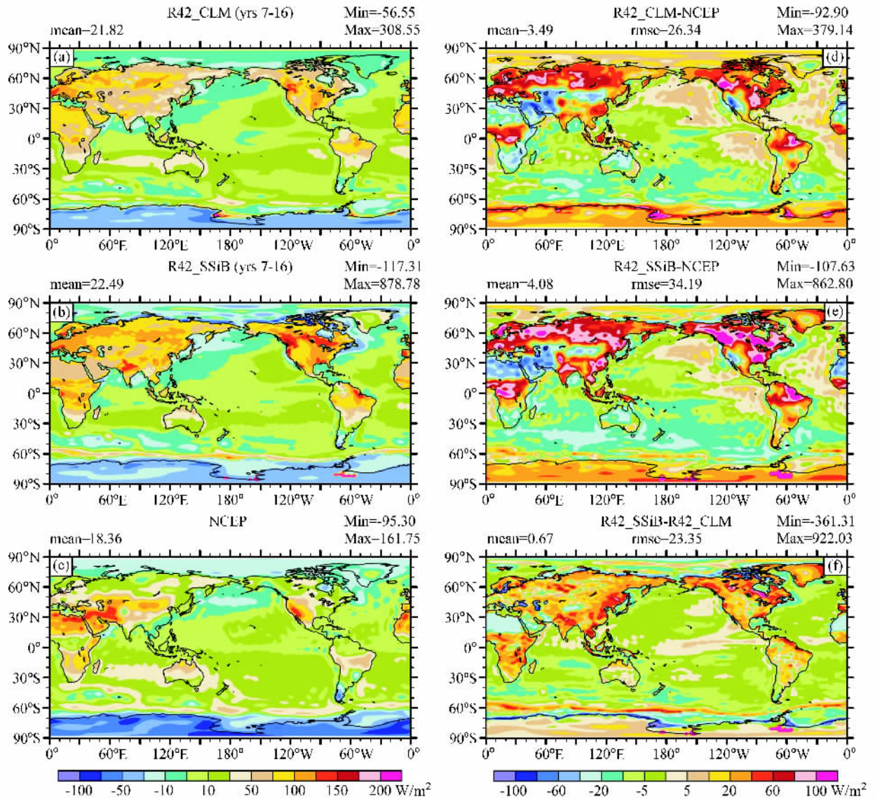
图2 R42_CLM (a)、R42_SSiB (b) 陆气耦合模式模拟和 NCEP 再分析 (c) 6~8 月 (JJA) 平均表面感热通量的全球平均分布以及它们之间的差异分布: (d) R42_CLM 与 NCEP 再分析资料的差异; (e) R42_SSiB 与 NCEP 再分析资料的差异; (f) R42_SSiB 与 R42_CLM 模式模拟差异。Min、Max、mean 和 rmse 分别表示最小值、最大值、平均值和均方根
