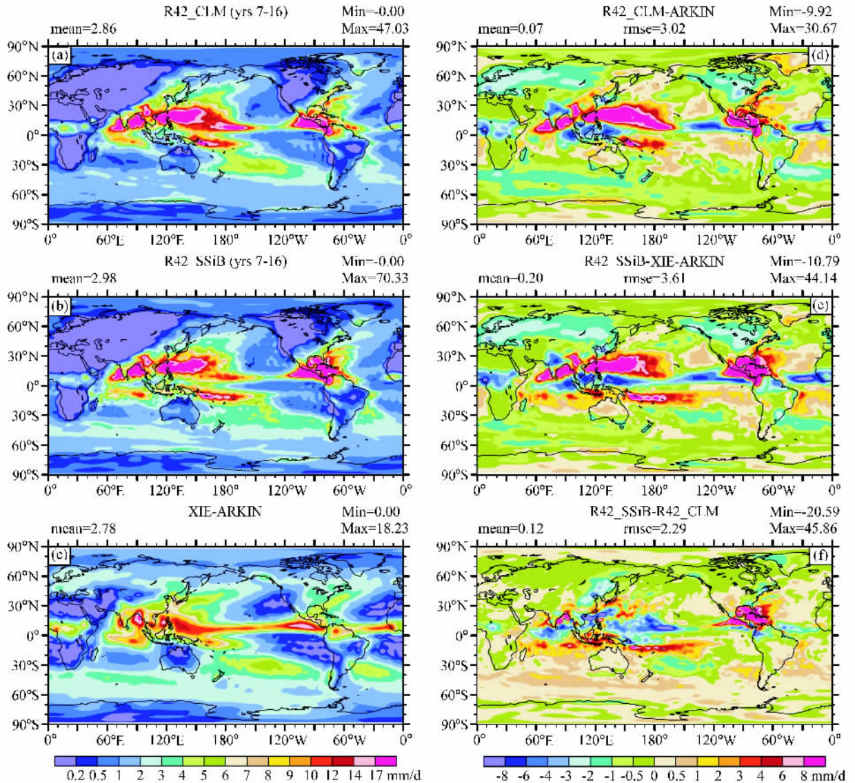
图 6 R42_CLM (a)、R42_SsiB (b) 陆气耦合模式模拟和 Xie-Arkin (c) 6~8 月 (JJA) 平均降水率的全球平均分布, 以及它们之间的差异分布: (d) R42_CLM 与 Xie-Arkin 资料的差异; (e) R42_SSiB 与 Xie-Arkin 资料的差异; (f) R42_SSiB 与 R42_CLM 模式模拟差异 Fig. 6 The JJA mean precipitation rates derived from R42_CLM (a), R42_SSiB (b), Xie-Arkin (c), and the differences between R42_CLM and Xie-Arkin (d), R42_SSiB and Xie-Arkin (e), and R42_SSiB and R42_CLM (f)
