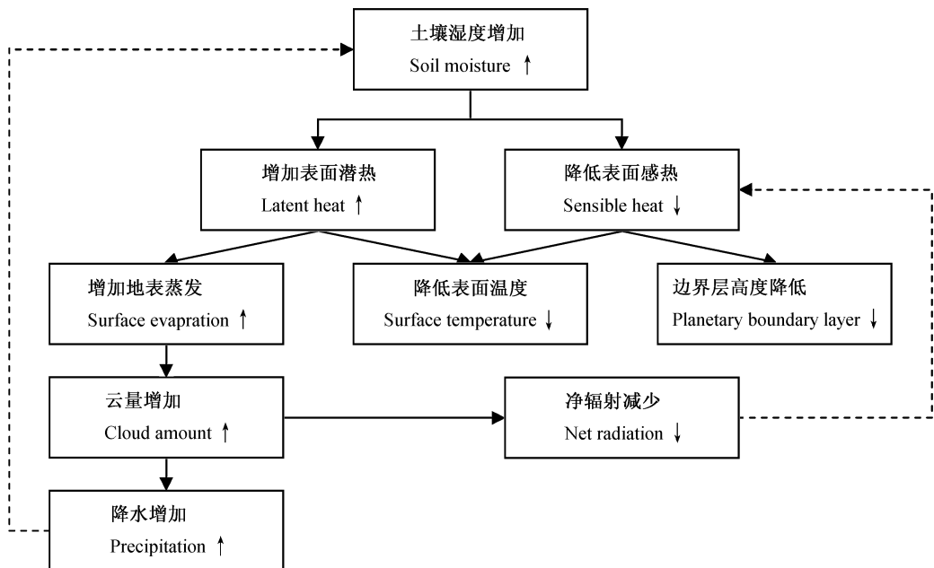
图 3 土壤湿度增加引起陆气通量变化的示意图(虚线表示正反馈过程)
