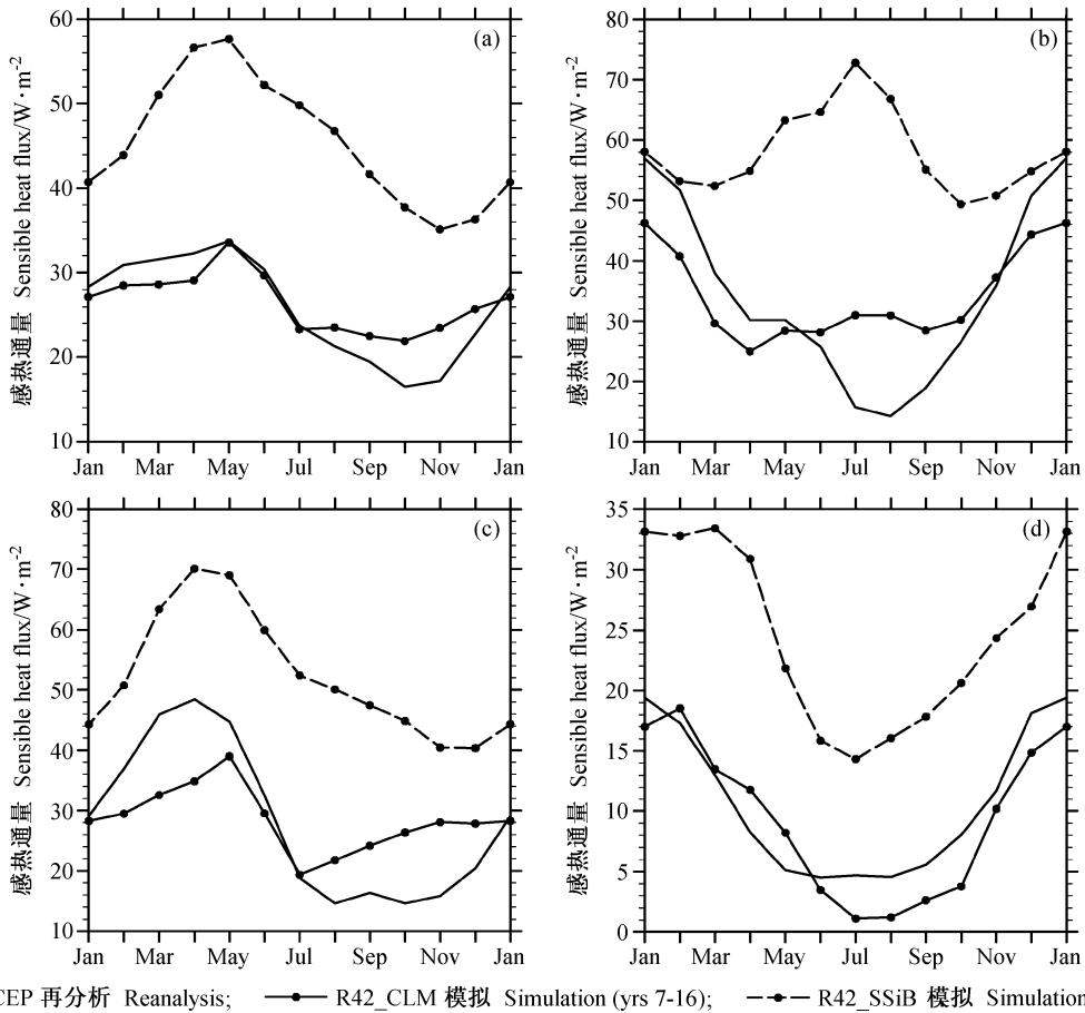
图 4 亚洲季风地区地表感热的季节演变: (a) 亚洲季风区 ( 5^{\circ}\text{N}\sim 45^{\circ}\text{N} , 60^{\circ}\text{E}\sim 150^{\circ}\text{E} ); (b) 东亚季风区 ( 22.5^{\circ}\text{N}\sim 45^{\circ}\text{N} , 100^{\circ}\text{E}\sim 140^{\circ}\text{E} ); (c) 印度季风区 ( 5^{\circ}\text{N}\sim 30^{\circ}\text{N} , 60^{\circ}\text{E}\sim 105^{\circ}\text{E} ); (d) 西北太平洋季风区 ( 5^{\circ}\text{N}\sim 22.5^{\circ}\text{N} , 105^{\circ}\text{E}\sim 150^{\circ}\text{E} )
