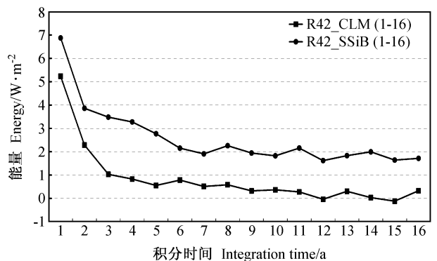
图 1 R42_CLM、R42_SSiB 陆气耦合模式所模拟全球平均地表面能量收支
