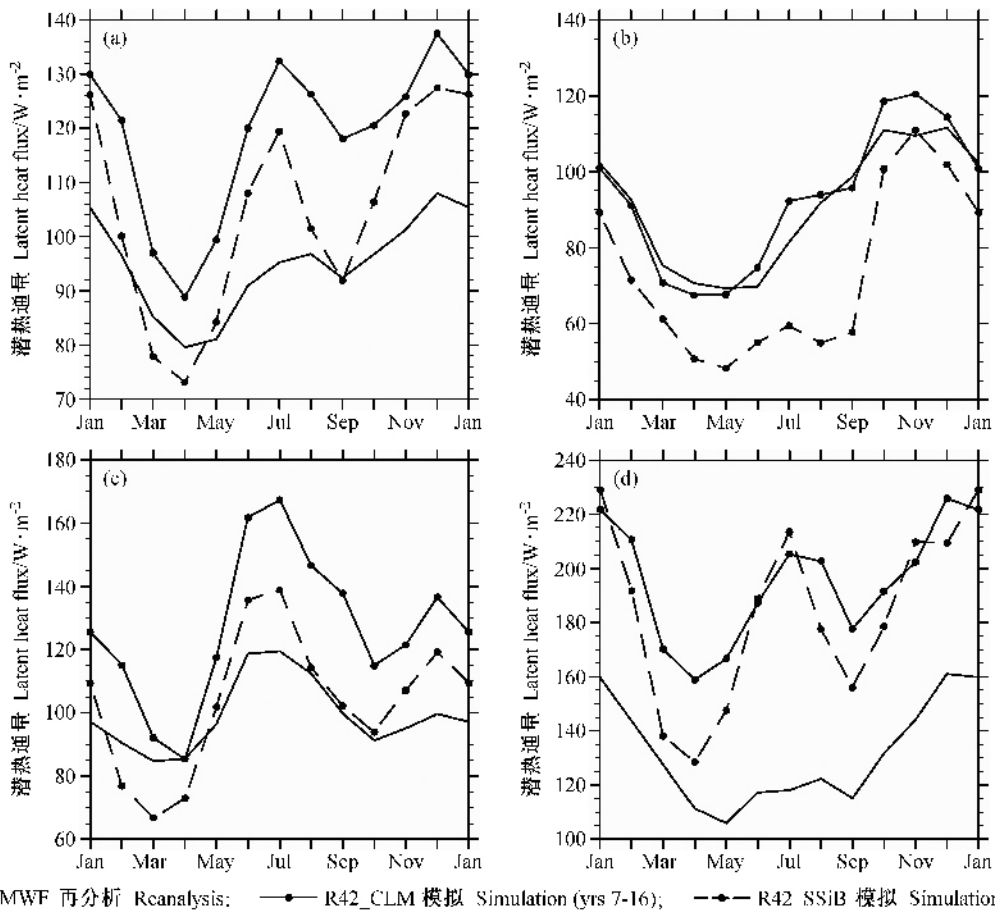
图 8 亚洲季风地区地表潜热的季节演变: (a) 亚洲季风区 ( 5^{\circ}\text{N}\sim 45^{\circ}\text{N} , 60^{\circ}\text{E}\sim 150^{\circ}\text{E} ); (b) 东亚季风区 ( 22.5^{\circ}\text{N}\sim 45^{\circ}\text{N} , 100^{\circ}\text{E}\sim 140^{\circ}\text{E} ); (c) 印度季风区 ( 5^{\circ}\text{N}\sim 30^{\circ}\text{N} , 60^{\circ}\text{E}\sim 105^{\circ}\text{E} ); (d) 西北太平洋季风区 ( 5^{\circ}\text{N}\sim 22.5^{\circ}\text{N} , 105^{\circ}\text{E}\sim 150^{\circ}\text{E} )
