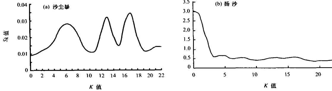
图 2 1954—1998 年沙尘暴与扬沙日数功率谱
